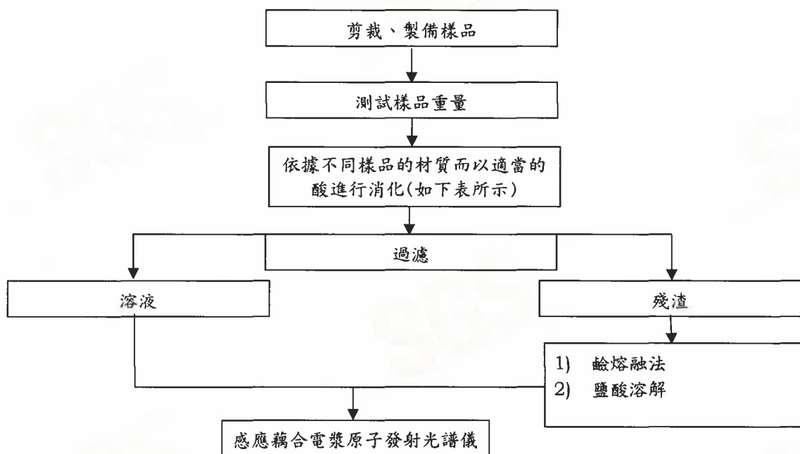
鎢、鉛的消化流程圖
